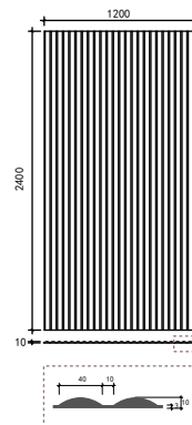
波浪-BL-003
