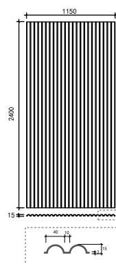
波浪-BL-002
