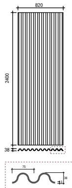
波浪-BL-001
