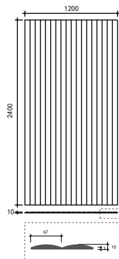
波浪-BL-001
